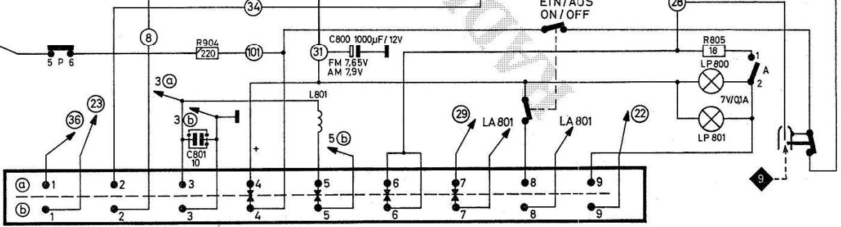
Umschaltsteckverbindung / Converting plug
