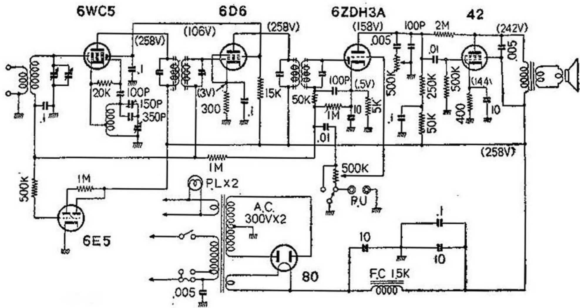
6 S 3 2 型受信機配線図
