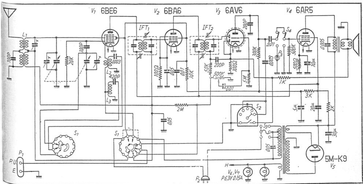
りぐいす ES の配線図
