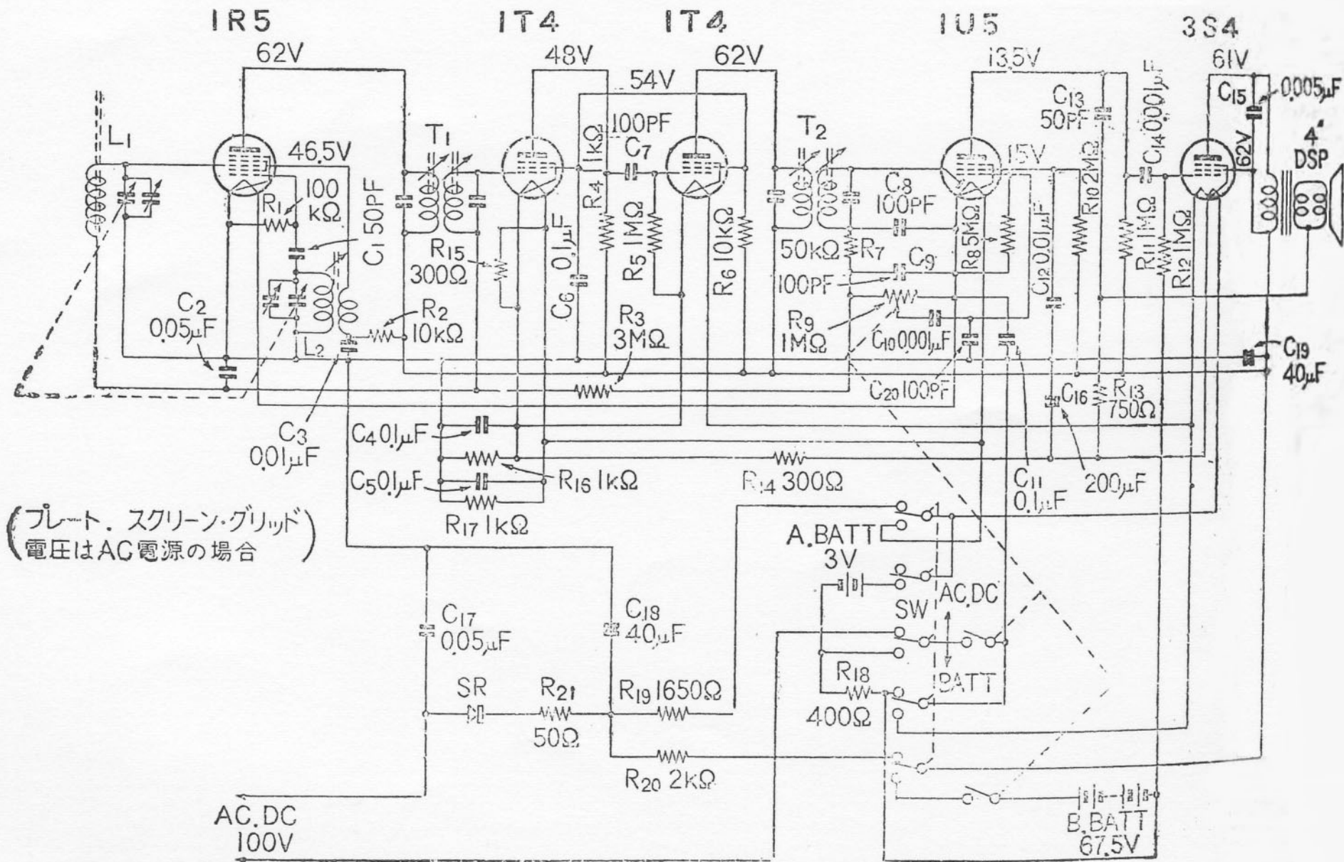
PS81 型受信機配線図
